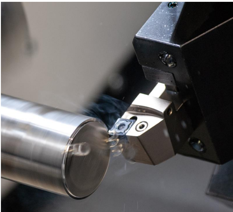
BU: Der Allrounder unter den Wendepplatten – die Hartmetallsorte PO41 15
